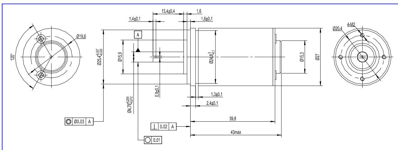
外形尺寸图
