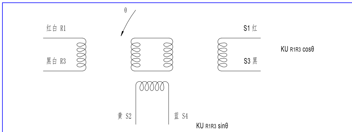
接线示意图
